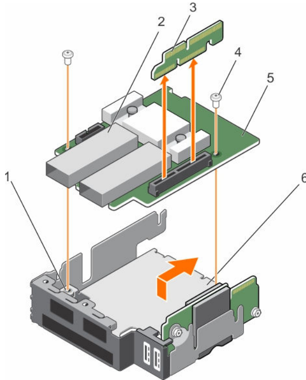
그림 16. PCIe 메자닌 카드 분리
