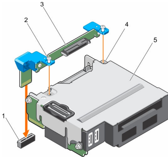
그림 41. SSD 후면판 설치
