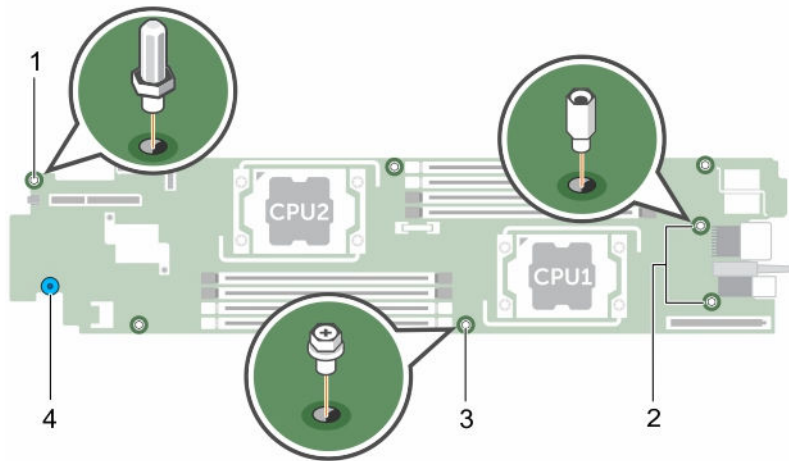
그림 44. 시스템 보드에 있는 나사 위치
