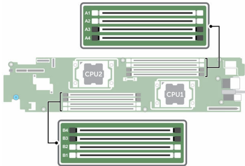
그림 12. 메모리 소켓 위치
