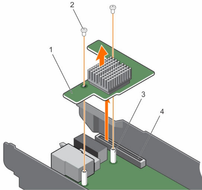
그림 24 . LOM 라이저 카드 분리
