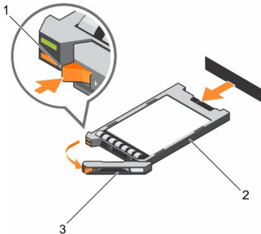
그림 34. SSD 캐리어 분리
