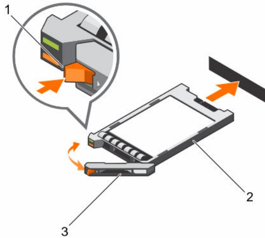
그림 35 . SSD 캐리어 설치
