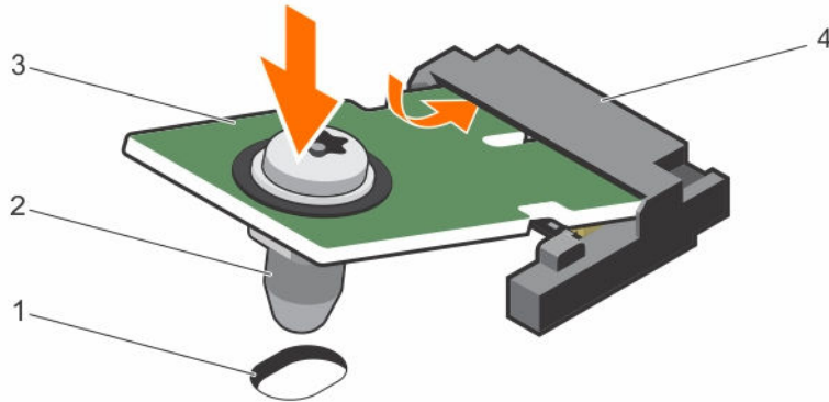
그림 47. TPM 설치
