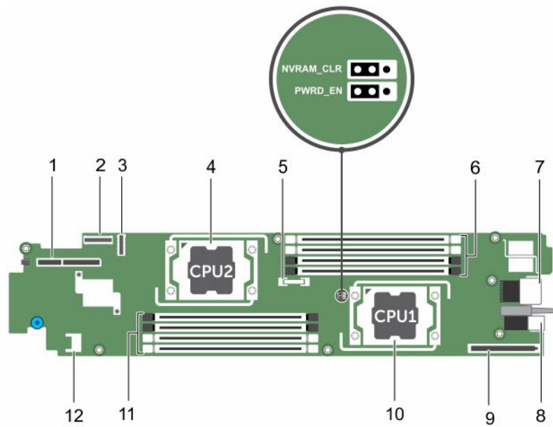
그림 48. 시스템 보드 커넥터
