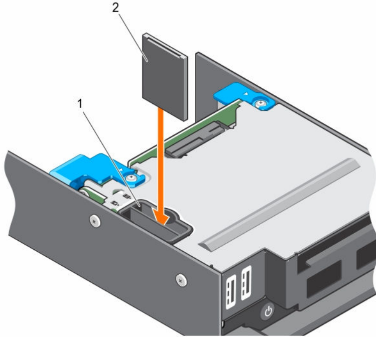
그림 19. 내부 SD 카드 설치
