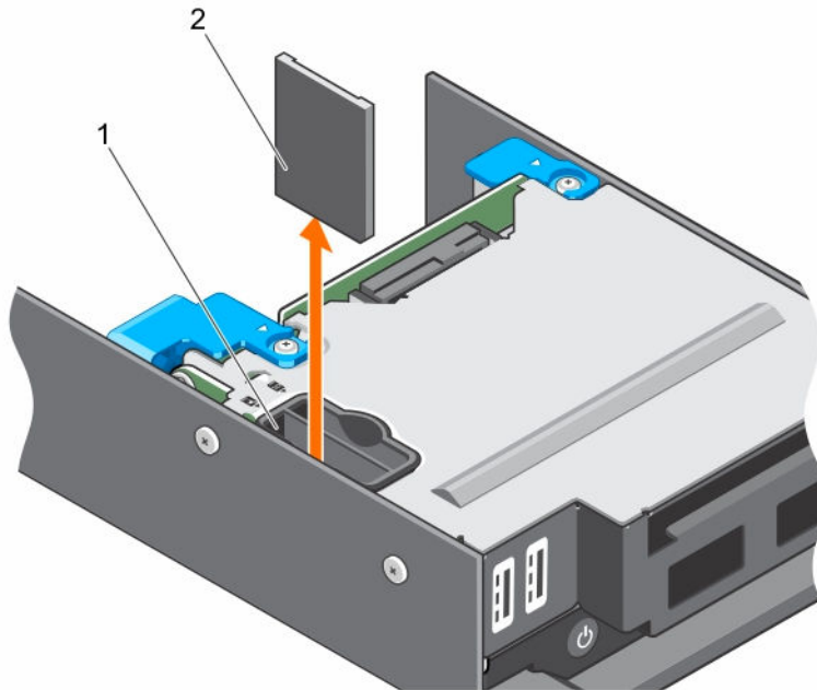
그림 22 . SD vFlash 카드 장착
