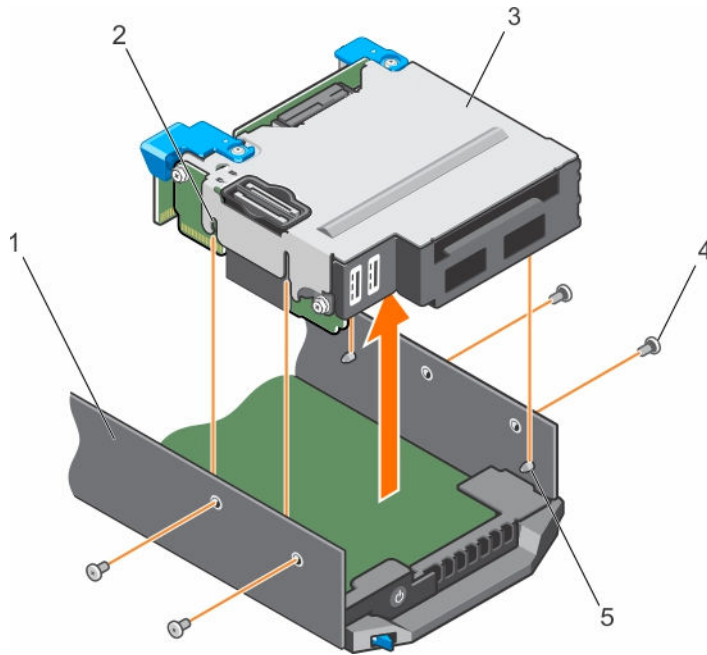
그림 38 . SSD 케이지 분리
