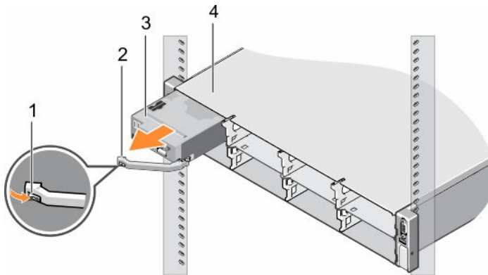
그림 7. 슬레드 분리
