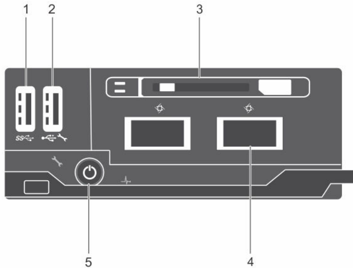
그림 2. 전면 패널 보기—단일 SSD 시스템
