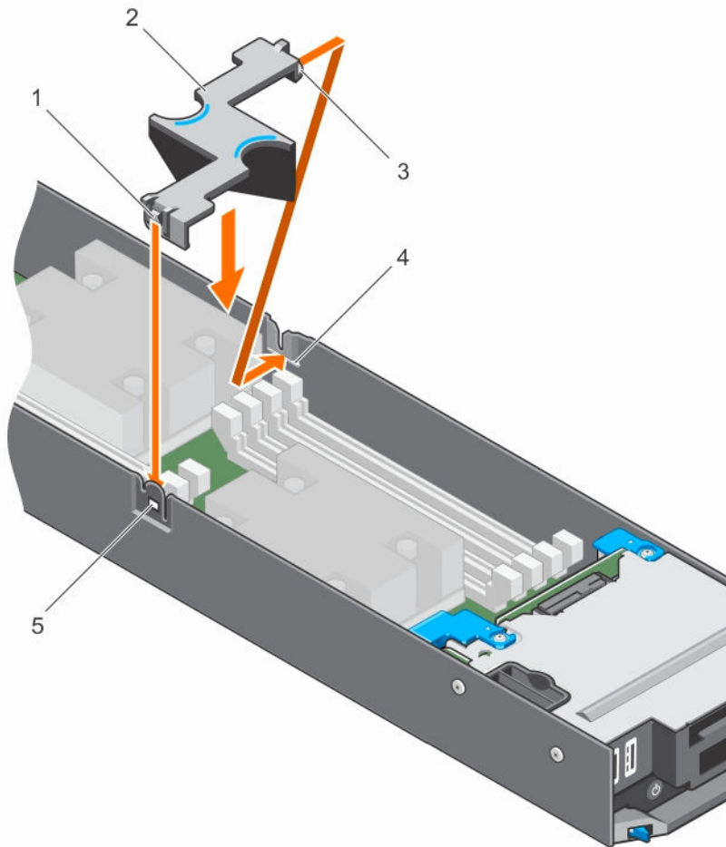
그림 11. 냉각 덮개 장착
