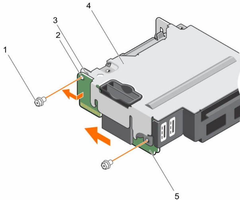
그림 20 . IDSDM 카드 제거
