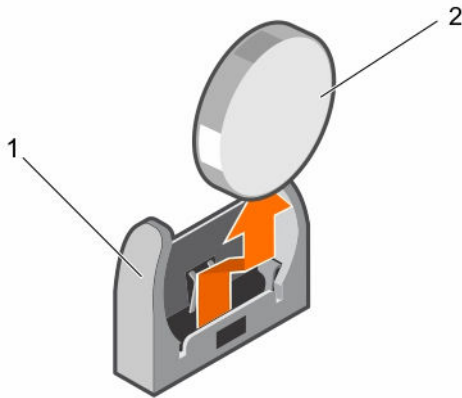
그림 42. NVRAM 백업 전지 문제 해결
