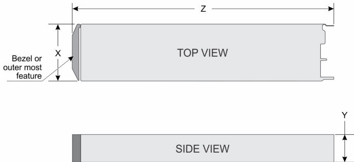
그림 6 . PowerEdge FC430 시스템의 새시 크기
