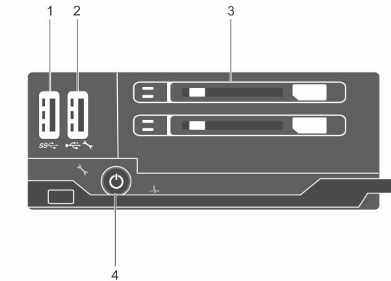
그림 3. 전면 패널 보기—이중 SSD 시스템
