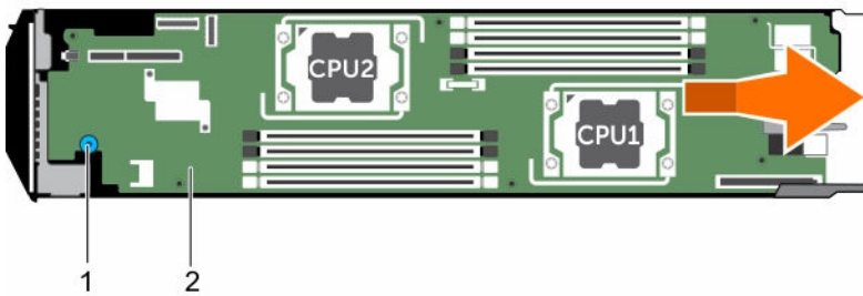
그림 45. 시스템 보드 제거
