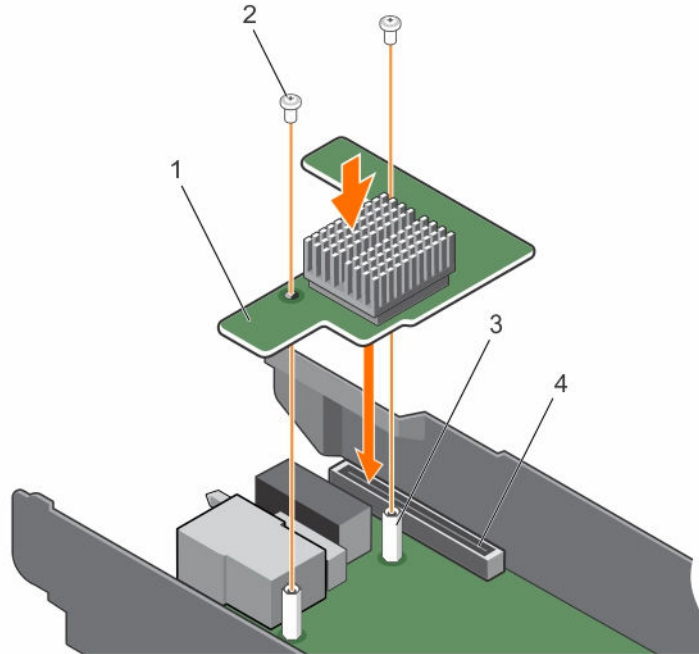
그림 25. LOM 라이저 카드 설치
