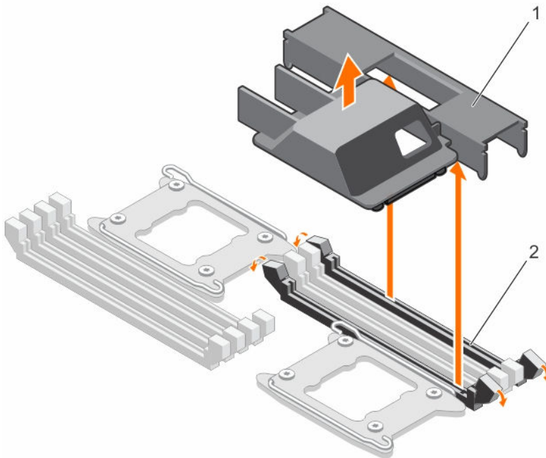
그림 31. 프로세서 보호물 및 DIMM 보호물 분리
