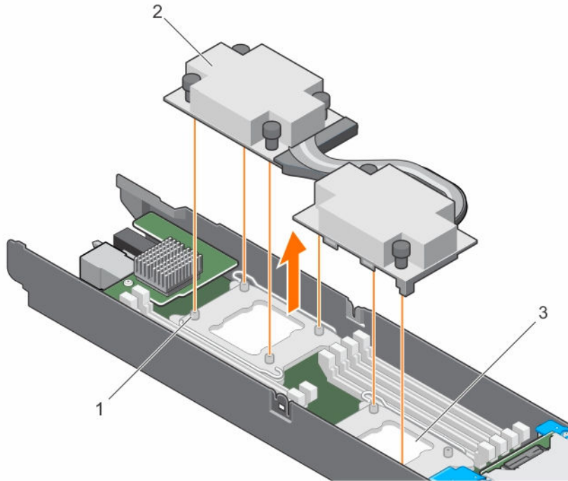
그림 27. 140W 방열판 분리
