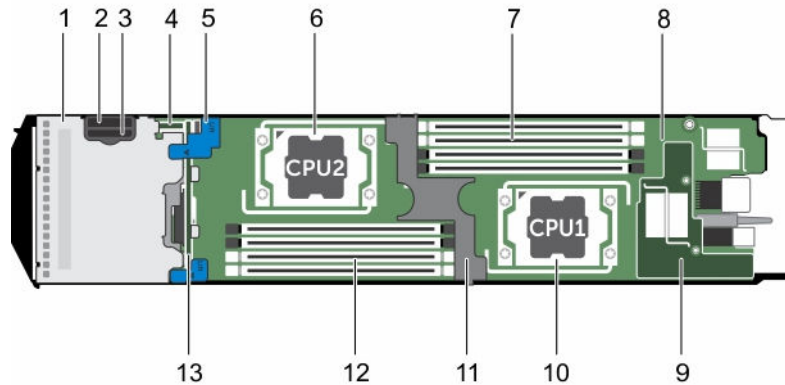
그림 9. 슬레드 내부
