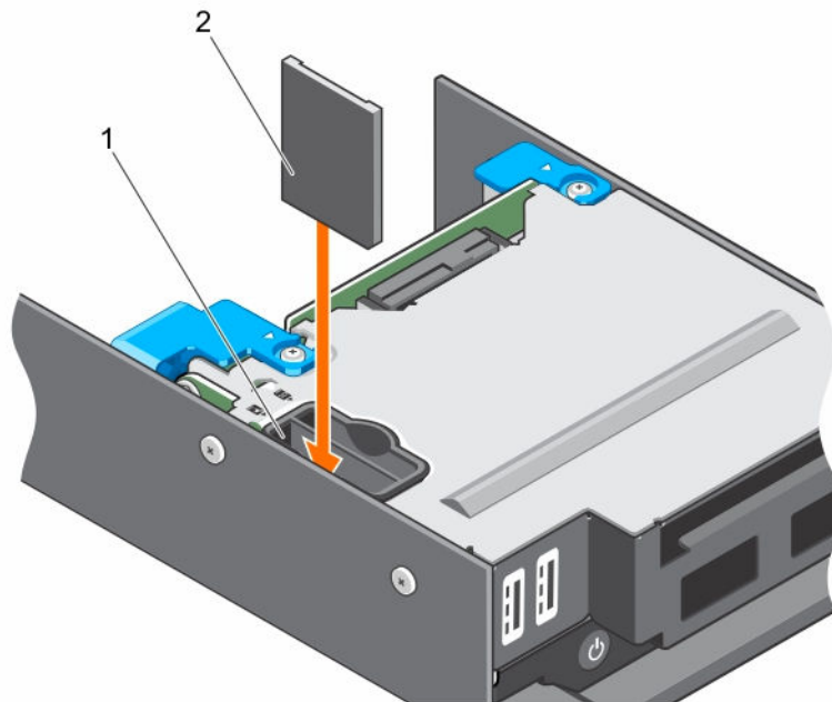
그림 23 . SD vFlash 카드 설치
