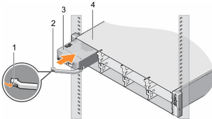
그림 8. 슬레드 설치
