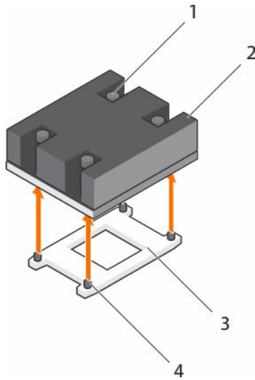
그림 26. 120W 방열판 분리
