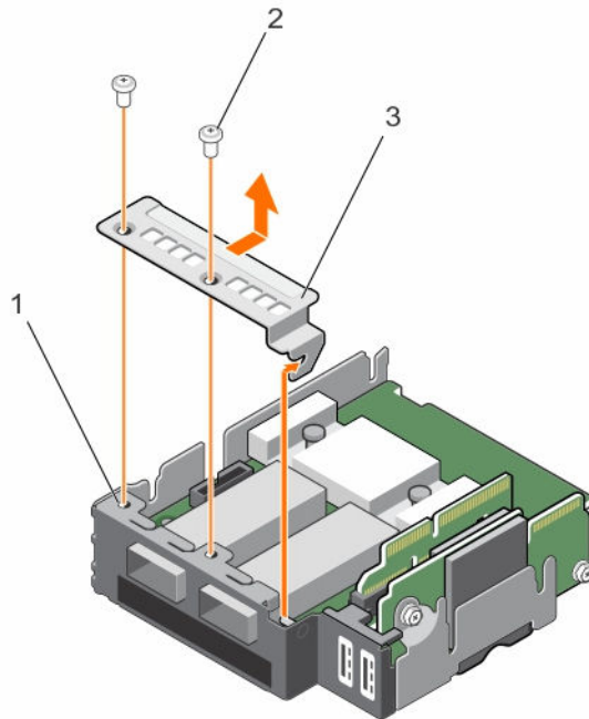
그림 15. SSD 케이스 베이스 덮개 제거
