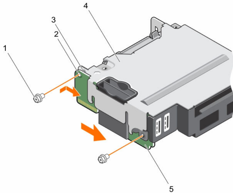
그림 21. IDSDM 카드 장착
