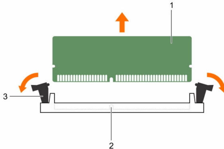
그림 13. 메모리 모듈 분리
