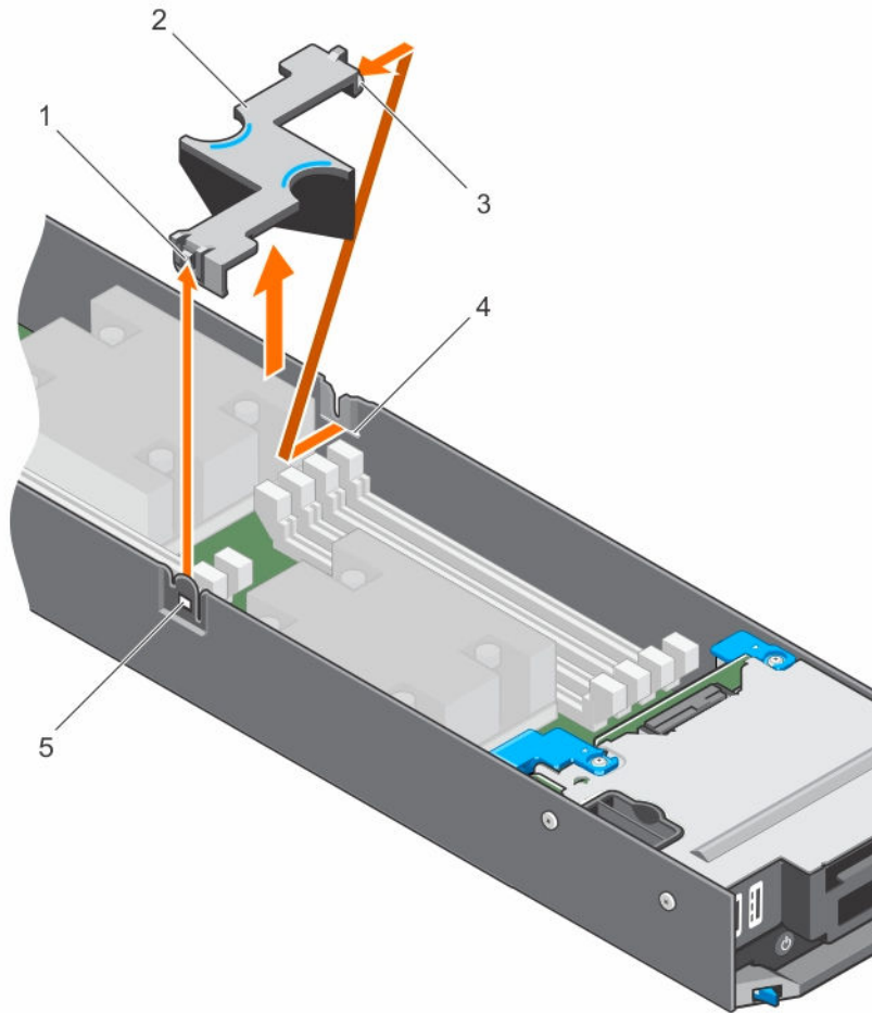
그림 10. 냉각 덮개 분리
