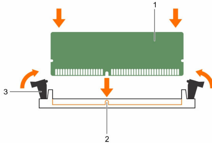
그림 14. 메모리 모듈 설치
