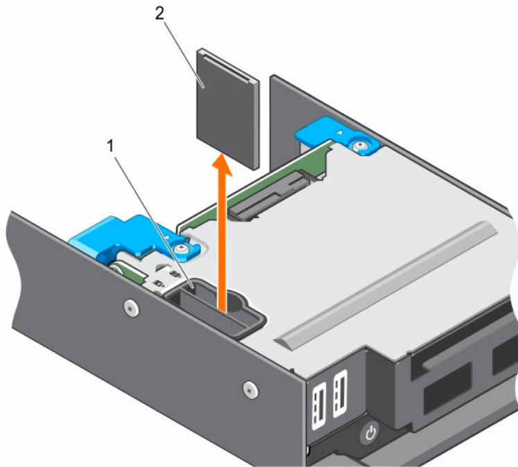
그림 18. 내부 SD 카드 장착
