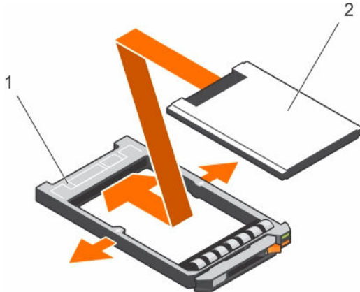
그림 33 . SSD 캐리어에 SSD 설치
