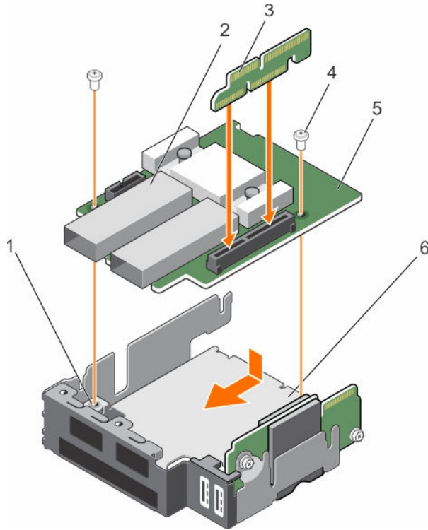
그림 17. PCIe 메자닌 카드 설치
