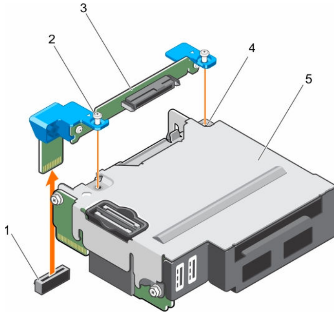
그림 40 . SSD 후면판 분리
